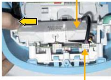
Złącze karty regulacji
