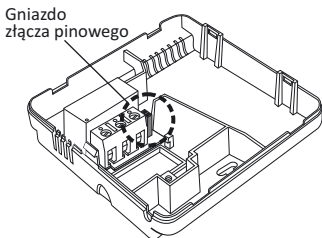
TYLNA OBUDOWA
